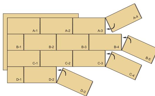
Схема установки панелей
